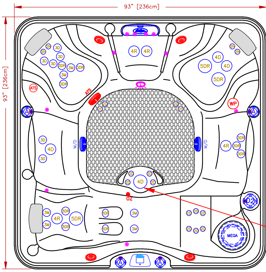
AAT (OPT20-AAT10) SEAT JET LAYOUT
